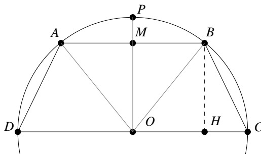
Figura 1.1: La soluzione a livello di scuola media: occorre sapere che, in questo caso, il trapezio è inscritto in una semicirconferenza.
