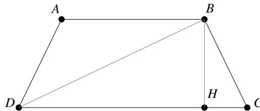
Figura 1.2: La soluzione a livello di scuola superiore: è sufficiente applicare il teorema di Pitagora a tre triangoli.
