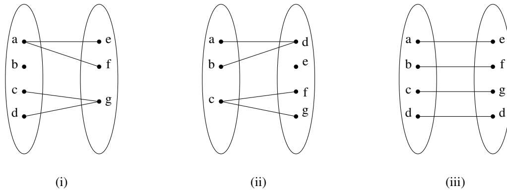
Figura 4.1: Le corrispondenze in (i) e (ii) sono esempi di corrispondenze non biunivoche. La corrispondenza in (iii) è biunivoca.
